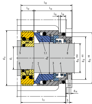
HRZ1
