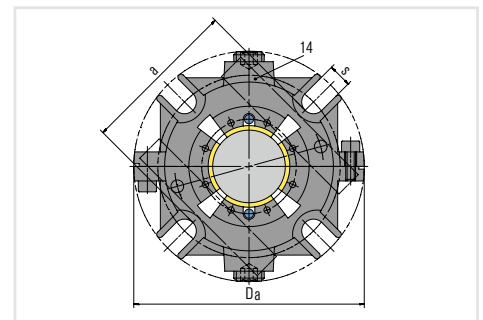
Dichtungsdeckel
