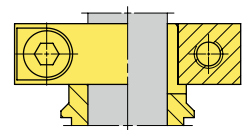
Klemmring
