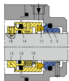
HJ4... (Beispiel)
