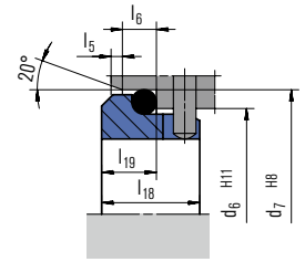
G16 (EN 12756)
