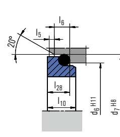
G6 EN 12756
