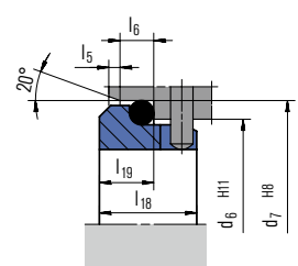
G16 (EN 12756)
