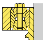
Spannsatz
