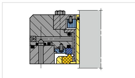
Spülung
