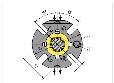
Dichtungsdeckel
