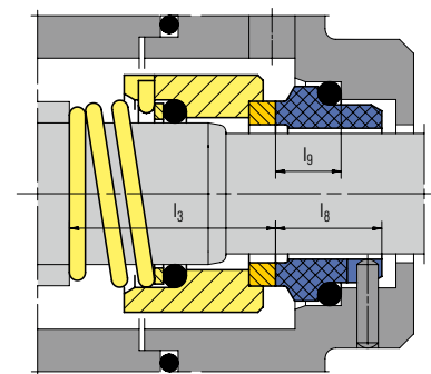
H176N
