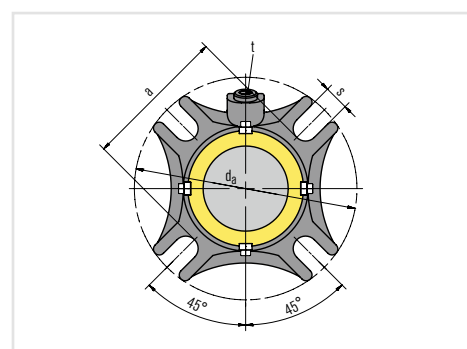
Dichtungsdeckel
